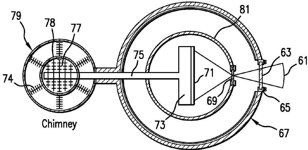
Solar Thermal Collector FIG. 10A
