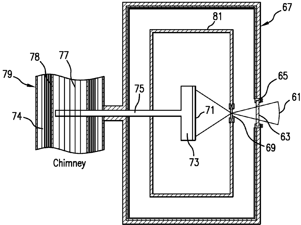
Solar Thermal Collector FIG. 10B
